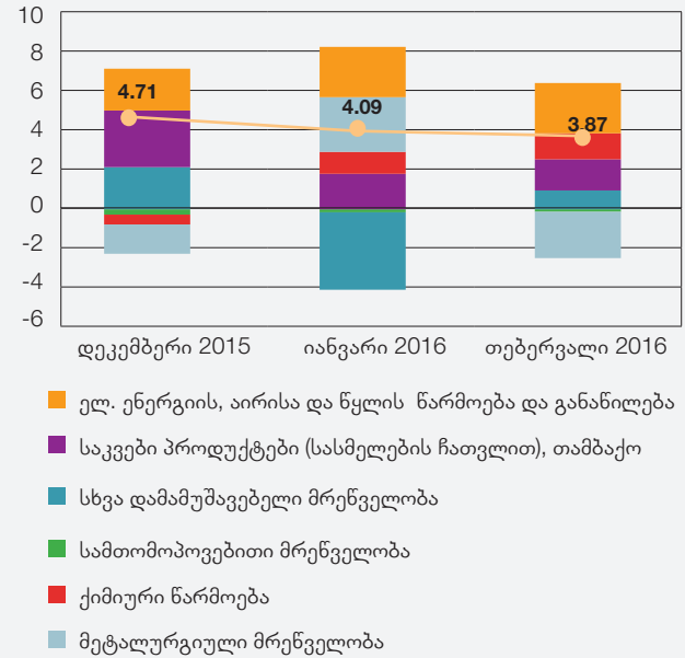
გრაფიკი 11: სამრეწველო პროდუქციის ფასების ინდექსის დეკომპოზიცია
